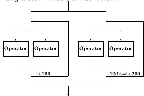
Abbildung 5: Parallelisierung einer Schleife mit in sich parallel laufenden Operatoren
