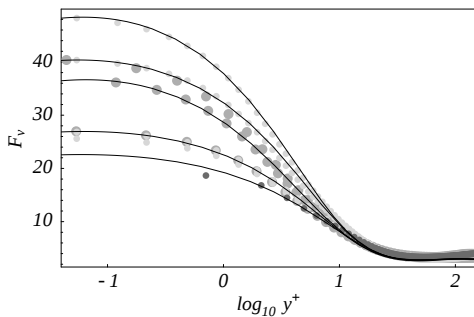
Abbildung 2: F_v -Profil aus Simulationen mit Lattice Boltzmann und Pseudospektralverfahren bei 178 \leq Re_\tau \leq 590 werden durch eine 4-Parameter Näherung der geraden Momente von v mit \log(y^+)^2 -Polynomen modelliert.
