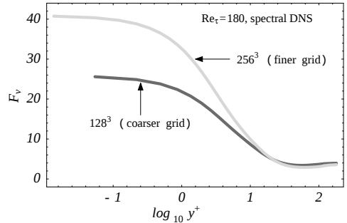
Abbildung 1: Voraussagen zweier numerischer Simulationen mit einem Pseudospektralverfahren jeweils verschiedener Auflösung, für die Abhängigkeit des Kurtosis F_v vom Wandabstand y^+ bei der Reynoldszahl Re_\tau = 180 .
