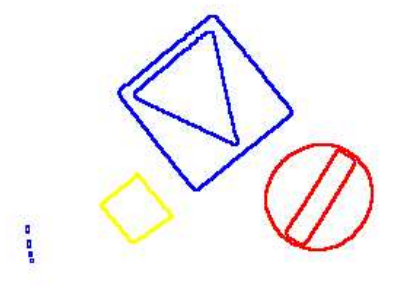
Abbildung 4: Farbsegmentierung
