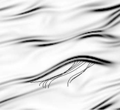
Abbildung 3: Destruktion Y_\epsilon , weiß/schwarz: niedrige/hohe Werte
