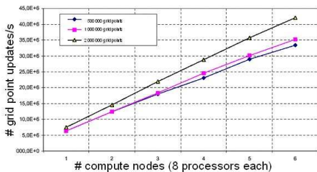
Abbildung 4: Leistungsmessung und Skalierung: Der Graph zeigt eine gute Skalierung des Problems auf der Hitachi SR8000, die auf die Parallelisierung über drei Ebenen (Vektorisierung, MPI- und SMP-Parallelisierung) zurückzuführen ist. Die Graphen wurden für unterschiedliche Gittergrößen gemessen und zeigen, dass sich die Parallelisierung über SMP und Vektorisierung noch mehr lohnt, je größer die Berechnungsgitter sind.
