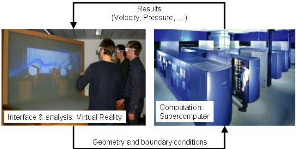
Abbildung 1: In dieser Abbildung wird der prinzipielle Datenfluss zwischen Holobench als Visualisierungs-Client und der Hitachi SR8000 auf der Simulationsseite gezeigt: In regelmäßigen Abständen wird die Änderung der Steuerparameter, Randbedingungen und Geometriedaten geprüft und gegebenenfalls vom VR-Interface zum Höchstleistungsrechner übertragen. Die Ergebnisse werden in benutzerdefinierten Zeitabständen an die Visualisierungskomponente gesendet. Dieser Kreislauf des Datenaustausches wird über die gesamte Laufzeit der Simulation fortgesetzt.
