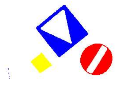
Abbildung 3: morphologische Operatoren
