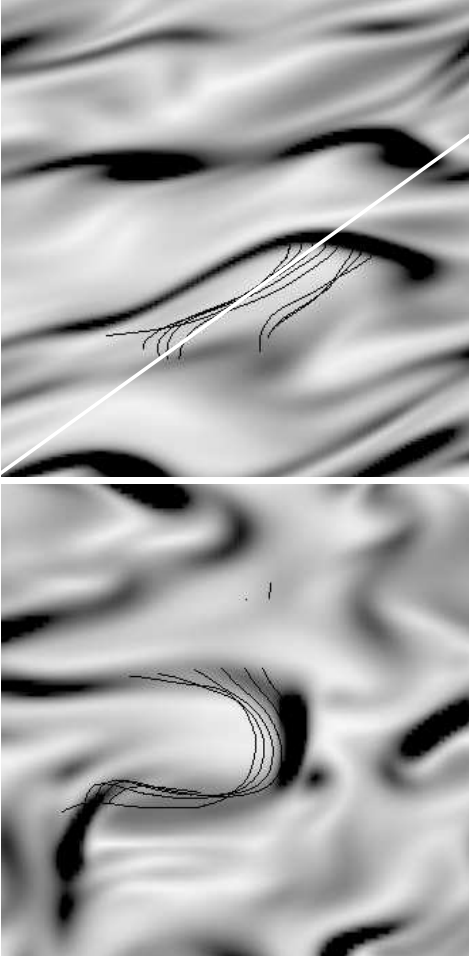
Abb. 1: Wirbelstärke \sqrt{\omega_i \omega_i} , weiß/schwarz: niedrige/hohe Intensität. Zusätzlich sind Wirbellinien eingezeichnet. Oben: Schnitt in spannweitischer Richtung, unten: Schnitt entlang der weißen Linie der oberen Abbildung.
