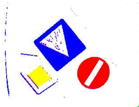
Abbildung 2: Farbklassifizierung
