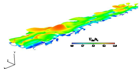
Abbildung 1: Isofläche der Wirbelstärke.
