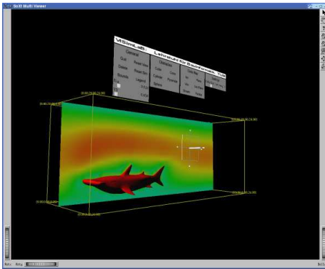
Abbildung 2: Als Beispiel einer komplexen CAD-generierten Geometrie wurde hier ein Hammerhai in das Fluidgebiet eingebracht.
