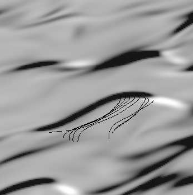
Abbildung 2: Produktion P_\epsilon^4 , weiß/schwarz: neg./pos. Werte
