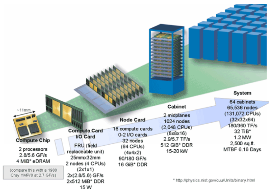
Abbildung 1: Schematischer Aufbau eines BlueGene/L Rechners
