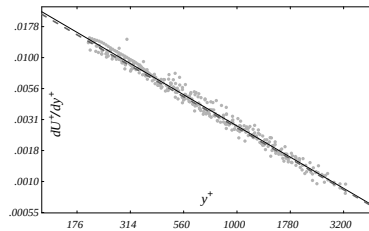
Abbildung 2: Logarithmisches Gesetz d\bar{U}/dy = \text{konst.}/y ; durchgezogen: beste Näherung \kappa = 0.362 , gestrichelt: \kappa = 1/e
