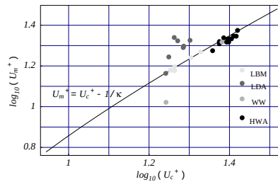
Abbildung 3: Asymptotische Genauigkeit (bei (U_m/u_\tau) \rightarrow \infty oder Re \rightarrow \infty ) von U_c/u_\tau \approx U_m/u_\tau + 1/\kappa .
